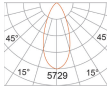
3000K- 24° BEAM
