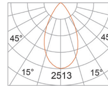
3000K- 41° BEAM
