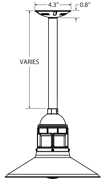
STEM MOUNT PENDANT (S)
