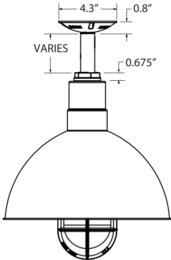
STEM MOUNT PENDANT (S)
