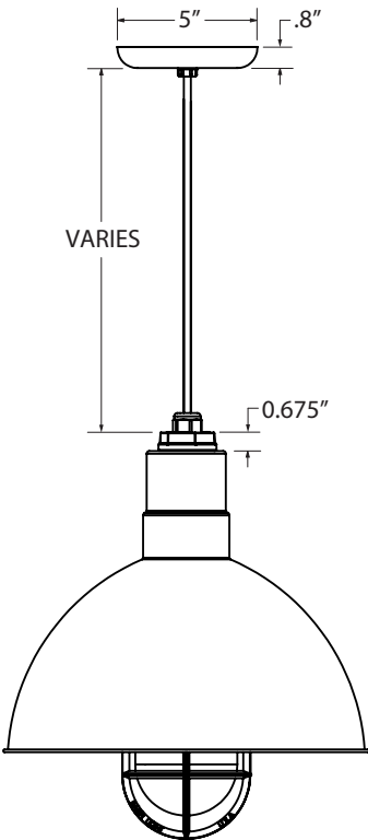
CORD HUNG PENDANT (C)
