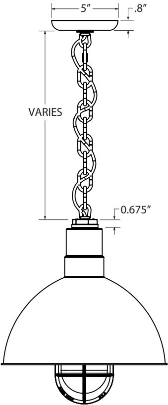
CHAIN HUNG PENDANT (CN)
