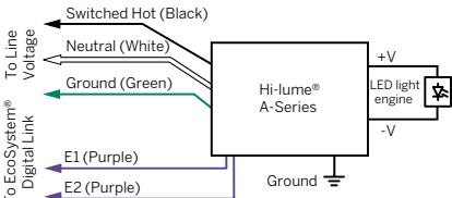
DES (Lutron 1% EcoSystem® digital)
