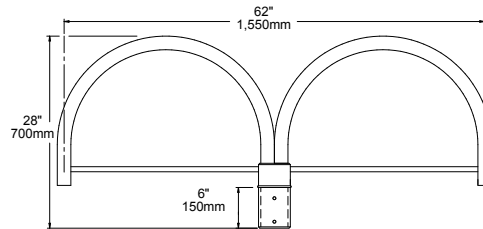
SLA18-2 (4" pole)
