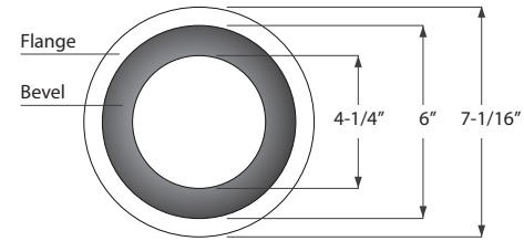
1 PIECE DIE CAST
